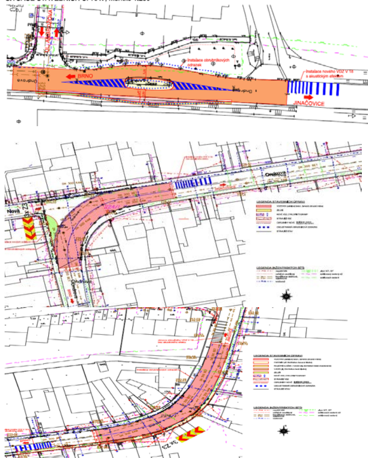
SITUACE STAVEBNÍCH ÚPRAV, měřítko 1:250
